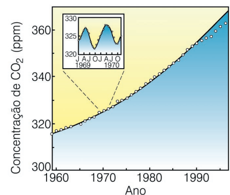
Figura 4: Variações na concentração do gás carbônico da troposfera determinadas pelo Laboratório de Oak Ridge em Mauna Loa, Hawaii. Extraída de Baird, 1998
