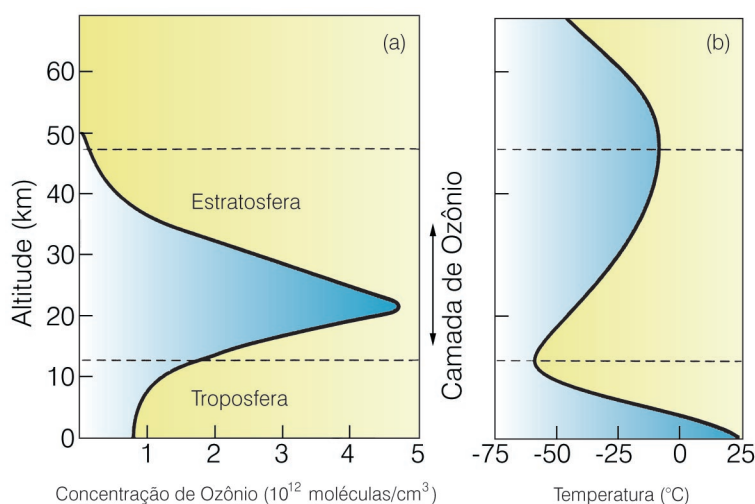
Figura 2: Variações da concentração de ozônio com a altitude para regiões de média latitude e da temperatura para a estratosfera e troposfera (Baird, 1998).
