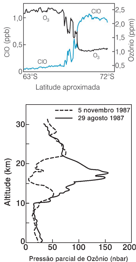
Figura 3: a. Concentração de ozônio e ClO em função da latitude no Pólo Sul. b. Distribuição vertical de ozônio no inverno (agosto) e primavera (novembro) de 1987 na Antártica (Baird, 1998).
